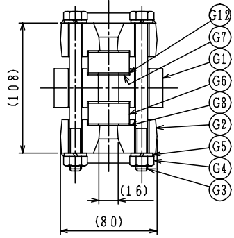
断面図 CROSS SECTION
