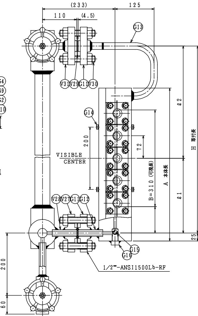
断面図 CROSS SECTION
